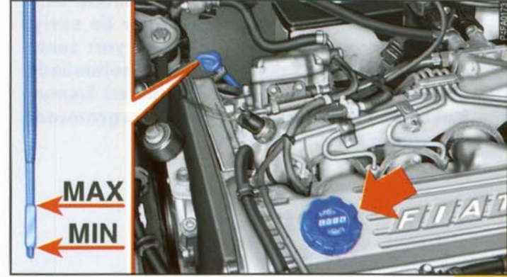
şekil 11 - 2.4 TD 125 tipi
