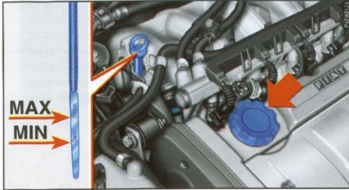
şekil 9 - 2.0 20V tipi
