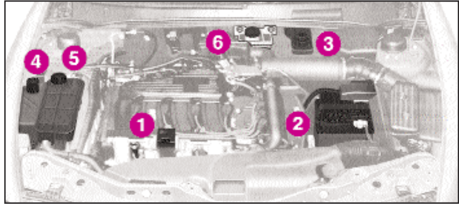
şekil 1 - 1.6 16V tipleri
