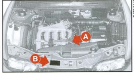
şekil 2 - 1.6 16V
