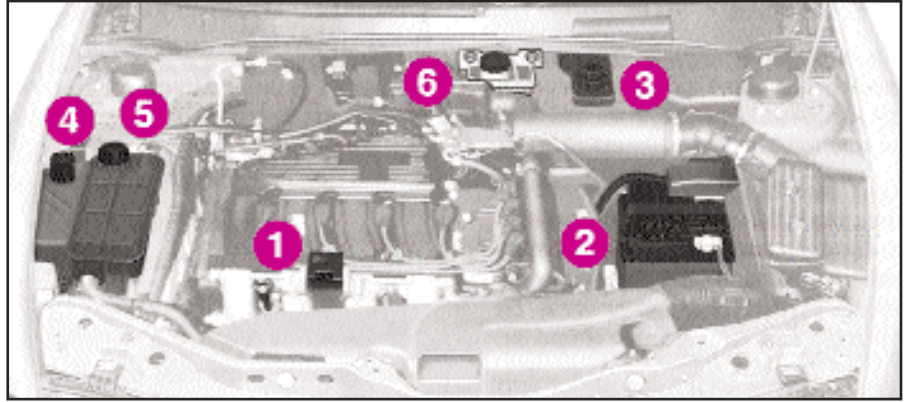
şekil 1 - 1.6 16v tipleri
